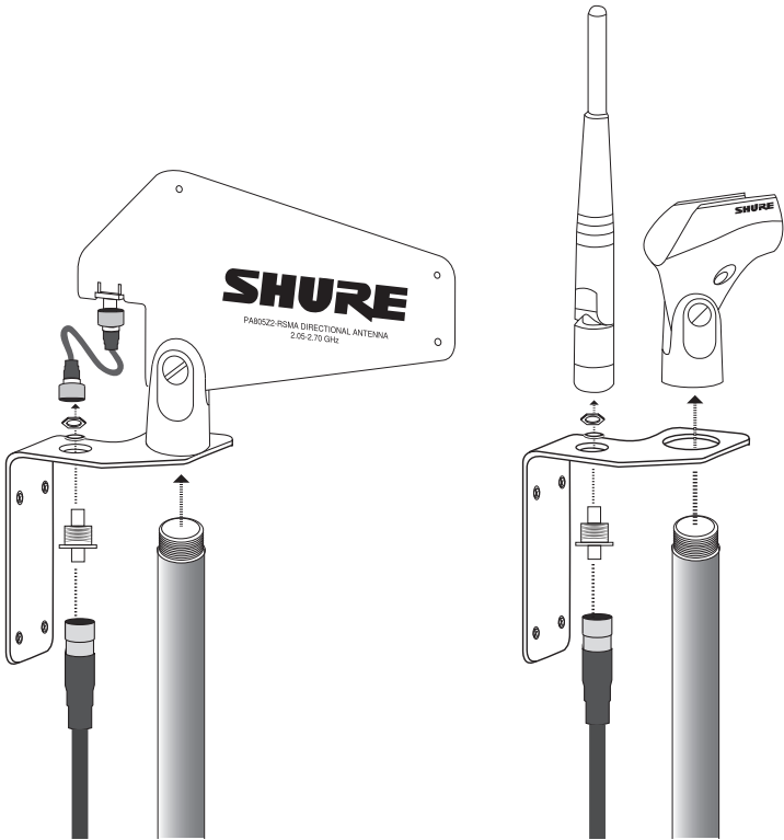
Mikrofonstativmontage
